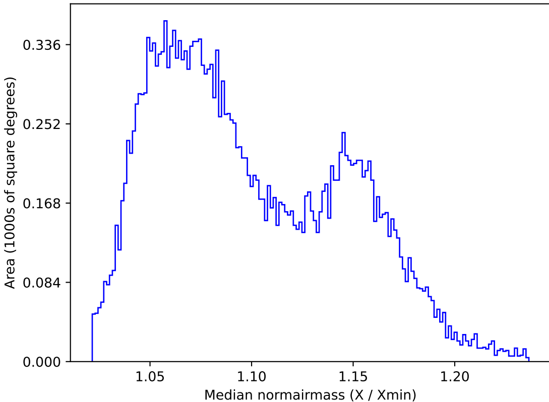
weather_cloudso6v3.4_10yrs All sky y band: Median normairmass
