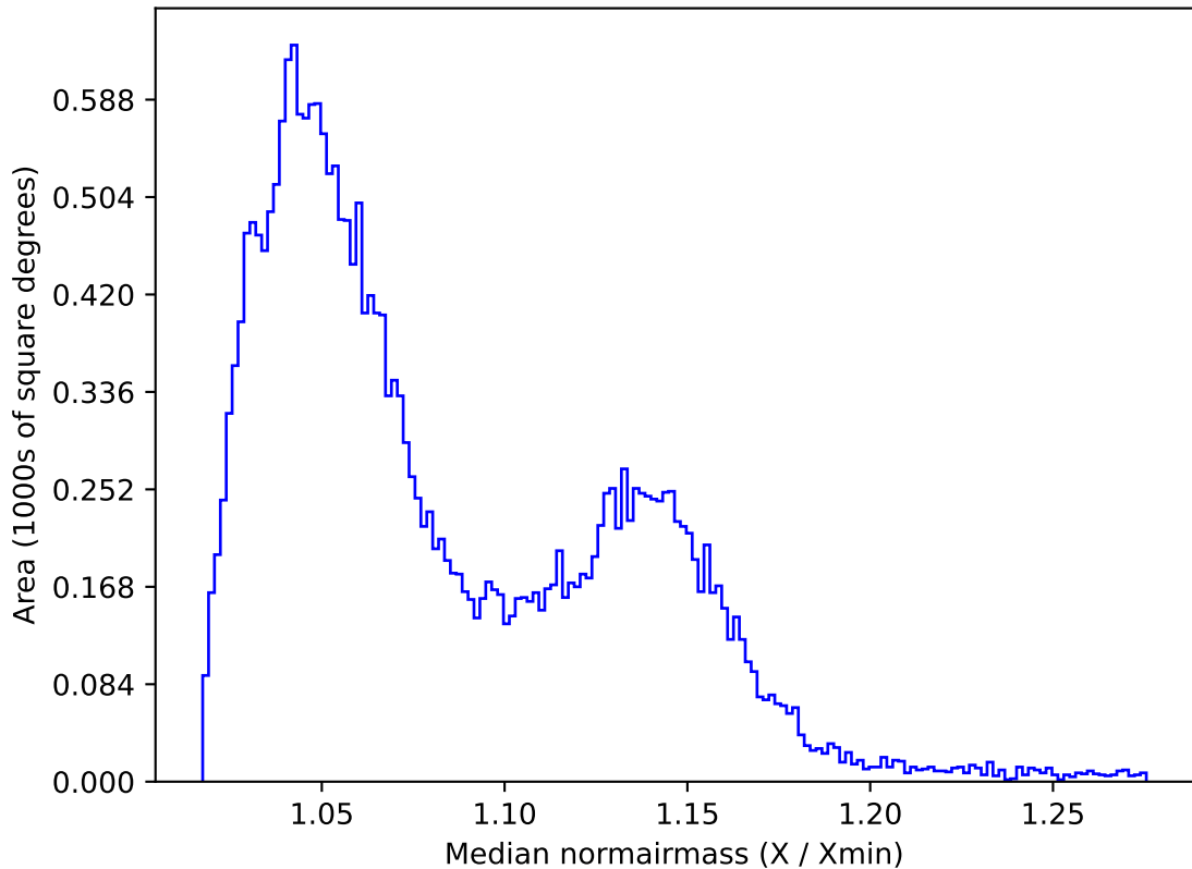
weather_cloudso6v3.4_10yrs All sky i band: Median normairmass
