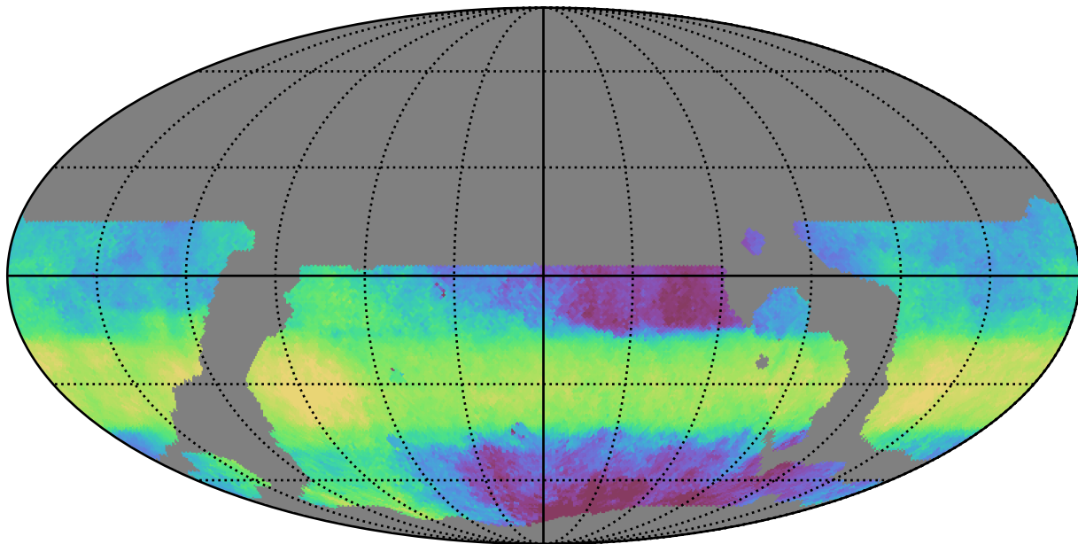
weather_cloudso6v3.4_10yrs WFD z band: Median HA
