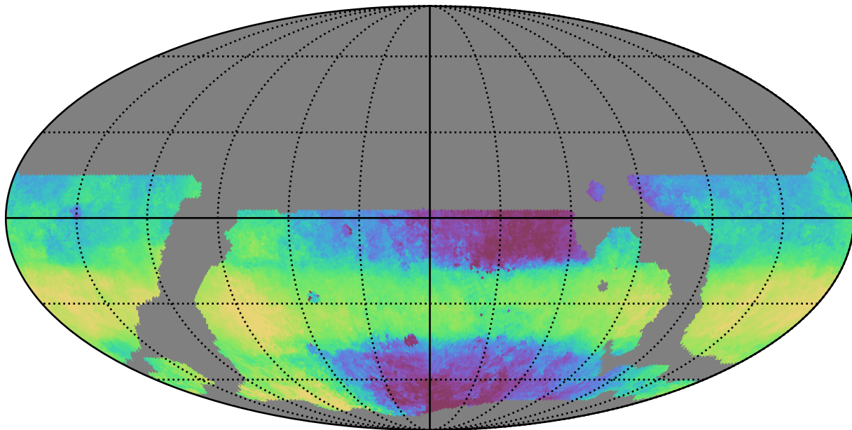
weather_cloudso6v3.4_10yrs WFD y band: Median HA
