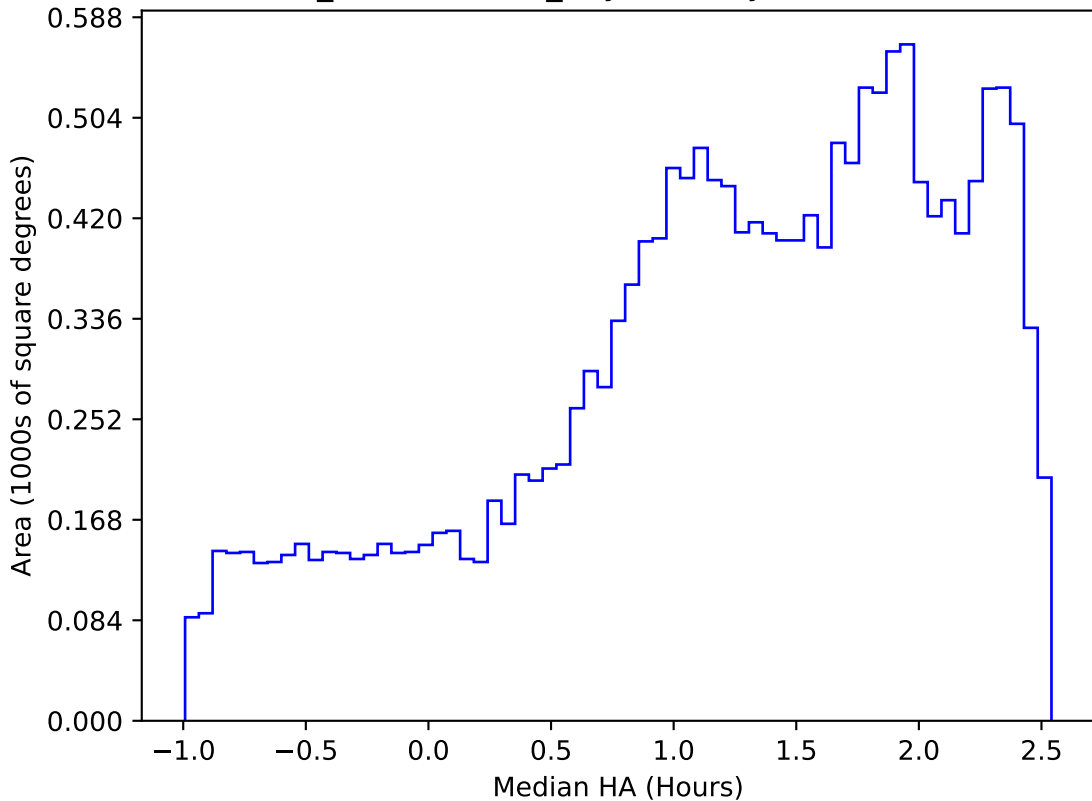
weather_cloudso6v3.4_10yrs WFD y band: Median HA
