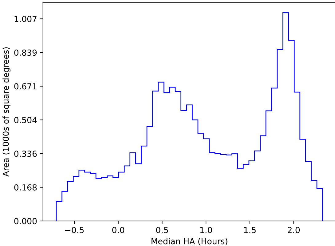
weather_cloudso6v3.4_10yrs WFD i band: Median HA
