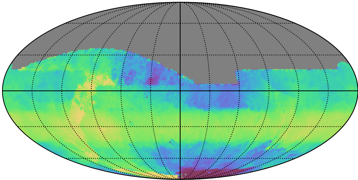
weather_cloudso6v3.4_10yrs All sky z band: Median HA
