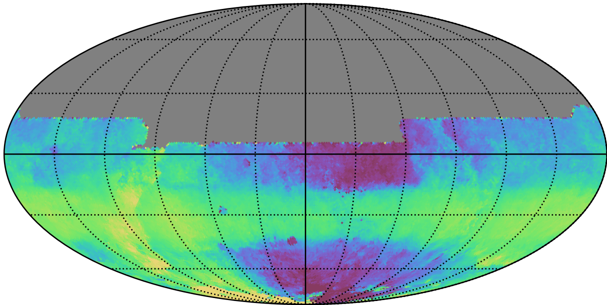
weather_cloudso6v3.4_10yrs All sky y band: Median HA
