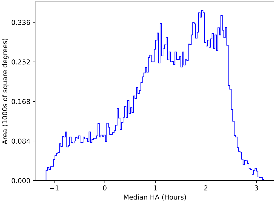
weather_cloudso6v3.4_10yrs All sky y band: Median HA
