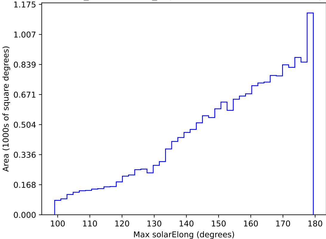
weather_cloudso6v3.4_10yrs WFD z band: Max solarElong
