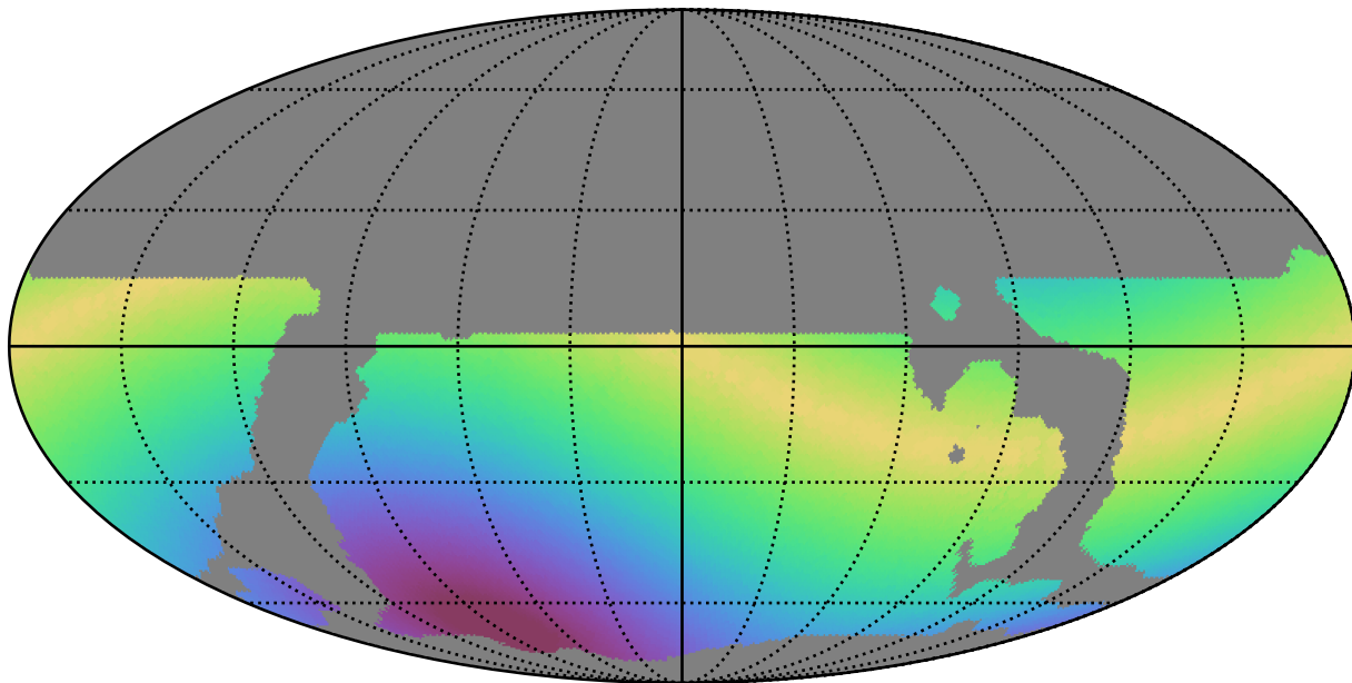
weather_cloudso6v3.4_10yrs WFD y band: Max solarElong
