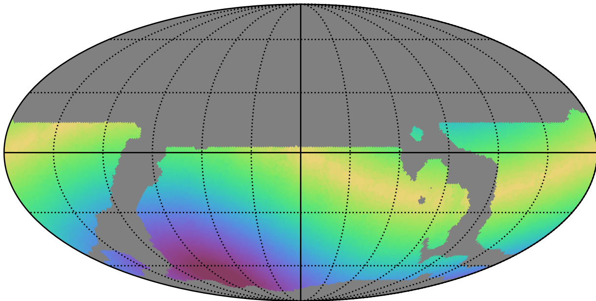
weather_cloudso6v3.4_10yrs WFD u band: Max solarElong
