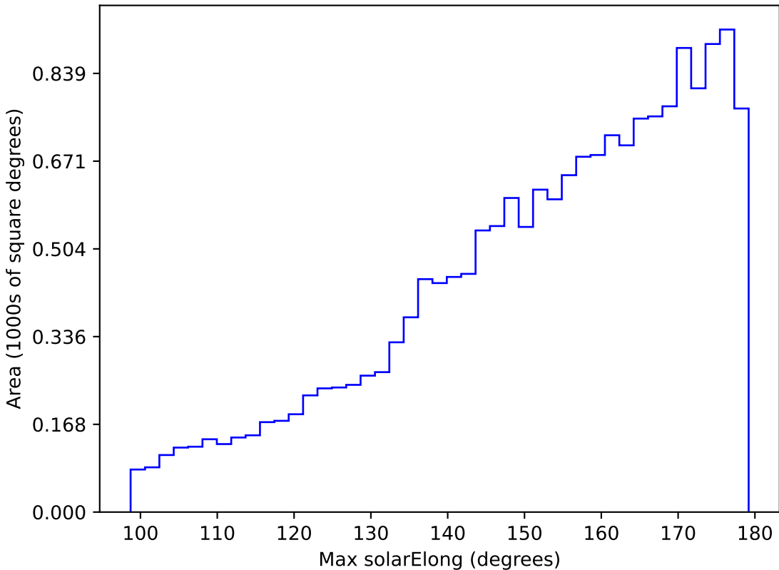
weather_cloudso6v3.4_10yrs WFD u band: Max solarElong
