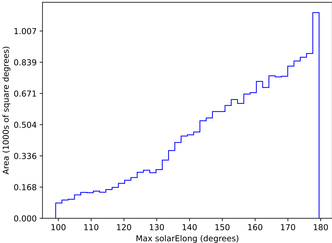
weather_cloudso6v3.4_10yrs WFD r band: Max solarElong
