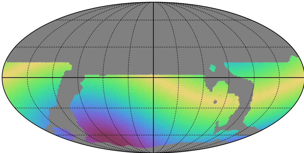
weather_cloudso6v3.4_10yrs WFD i band: Max solarElong
