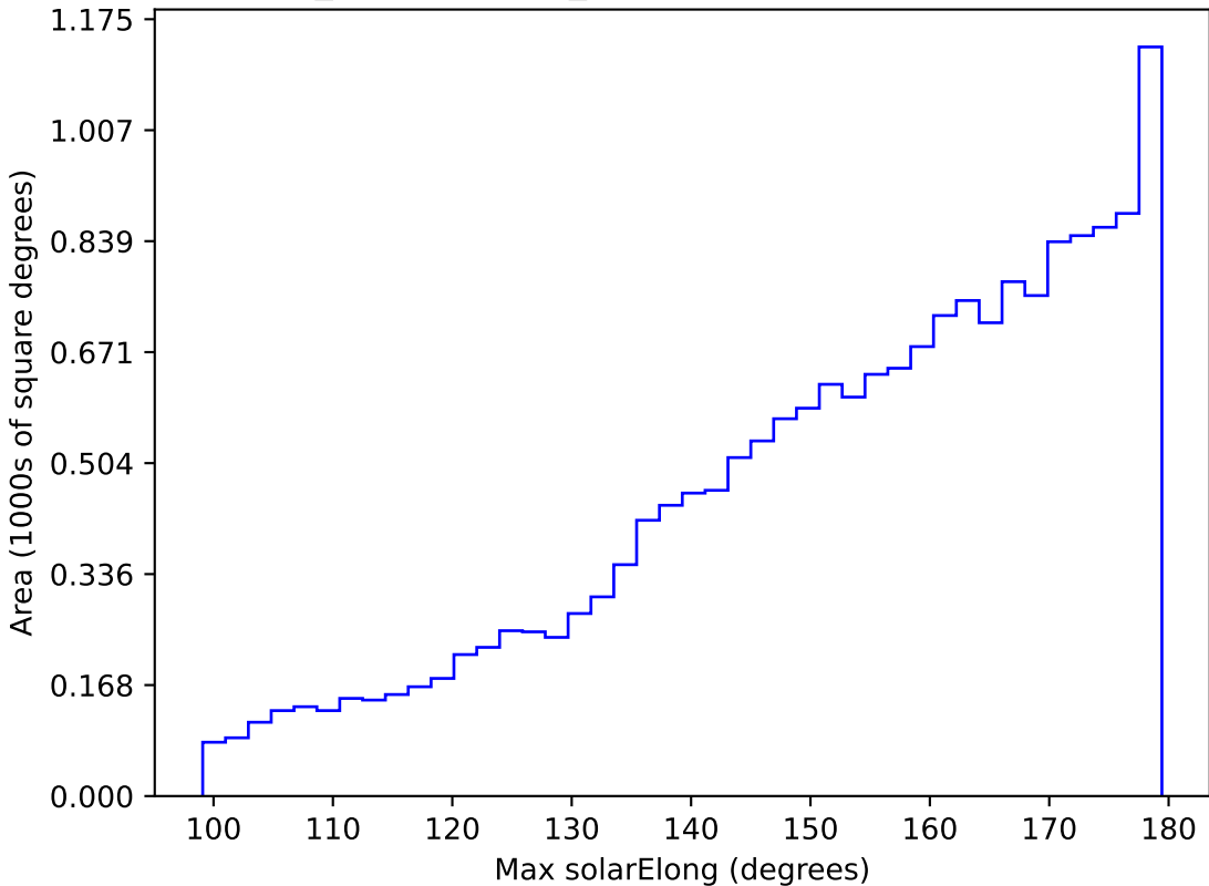
weather_cloudso6v3.4_10yrs WFD i band: Max solarElong
