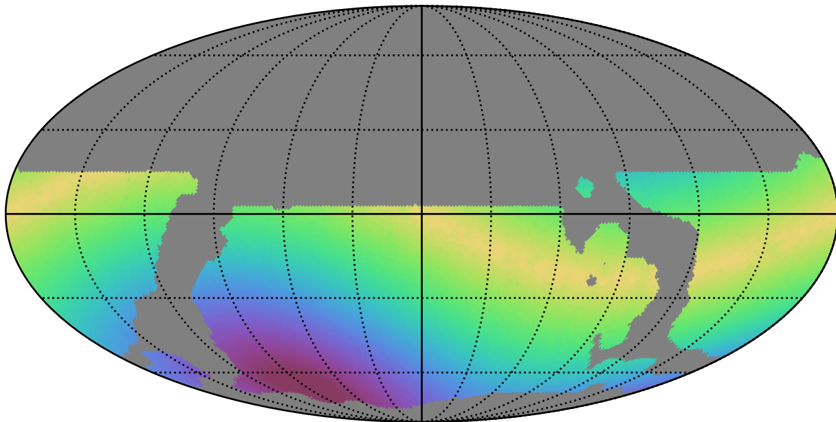
weather_cloudso6v3.4_10yrs WFD g band: Max solarElong
