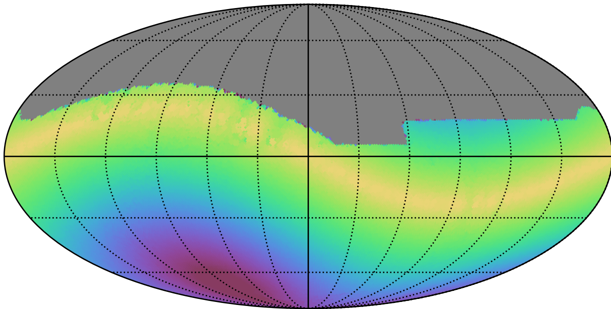
weather_cloudso6v3.4_10yrs All sky z band: Max solarElong
