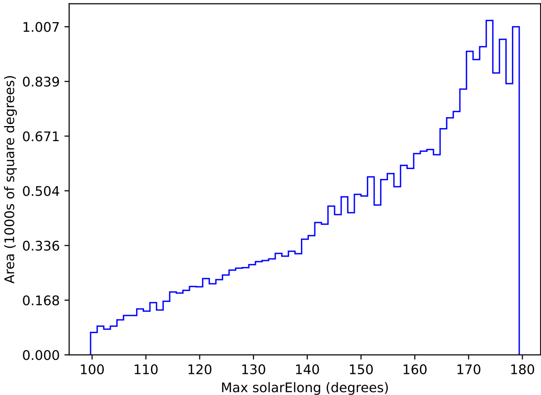
weather_cloudso6v3.4_10yrs All sky z band: Max solarElong
