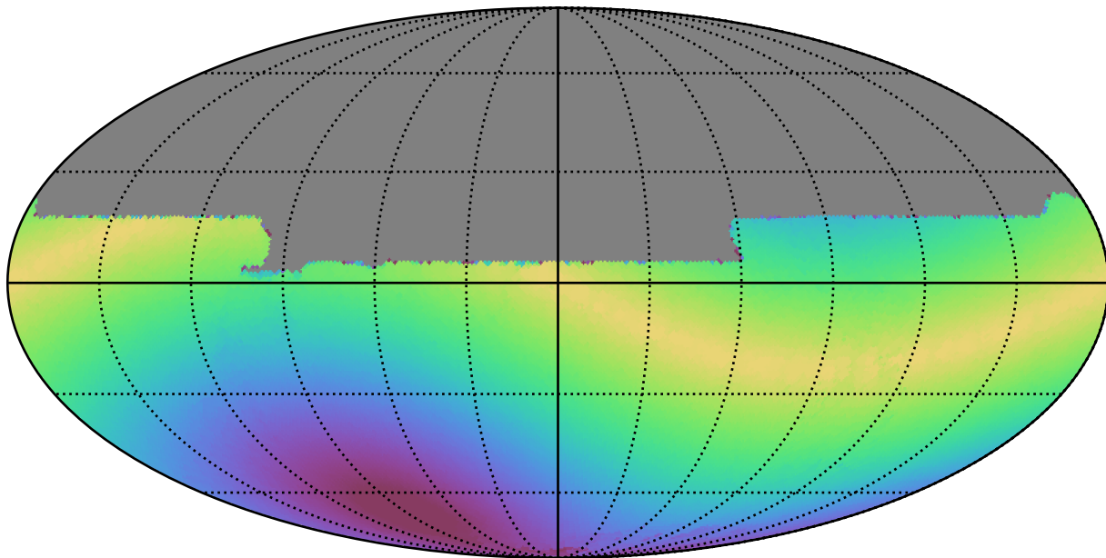
weather_cloudso6v3.4_10yrs All sky y band: Max solarElong
