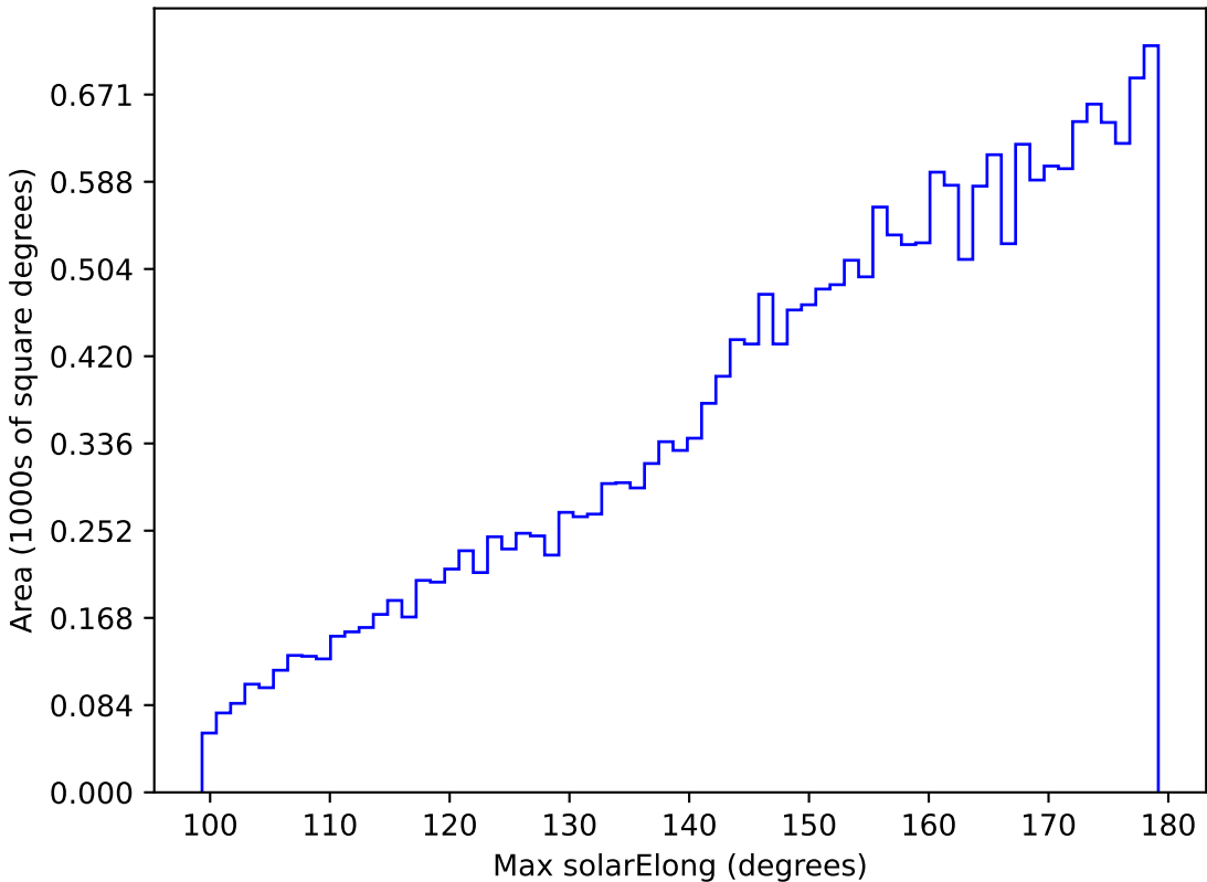
weather_cloudso6v3.4_10yrs All sky y band: Max solarElong
