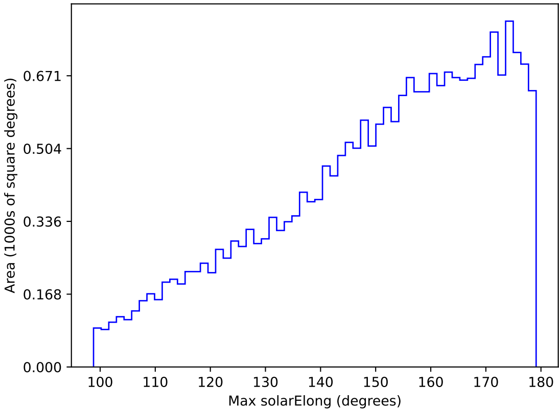
weather_cloudso6v3.4_10yrs All sky u band: Max solarElong
