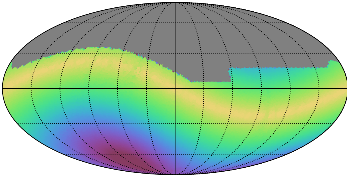
weather_cloudso6v3.4_10yrs All sky i band: Max solarElong
