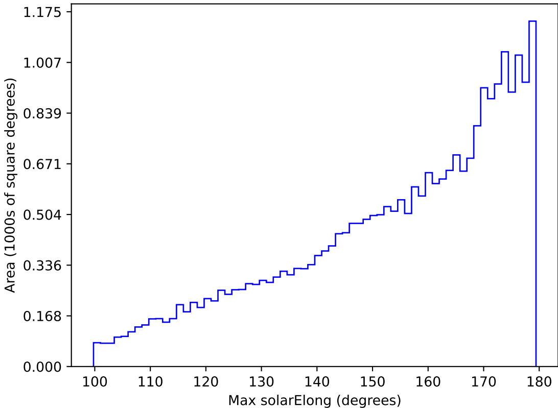
weather_cloudso6v3.4_10yrs All sky i band: Max solarElong
