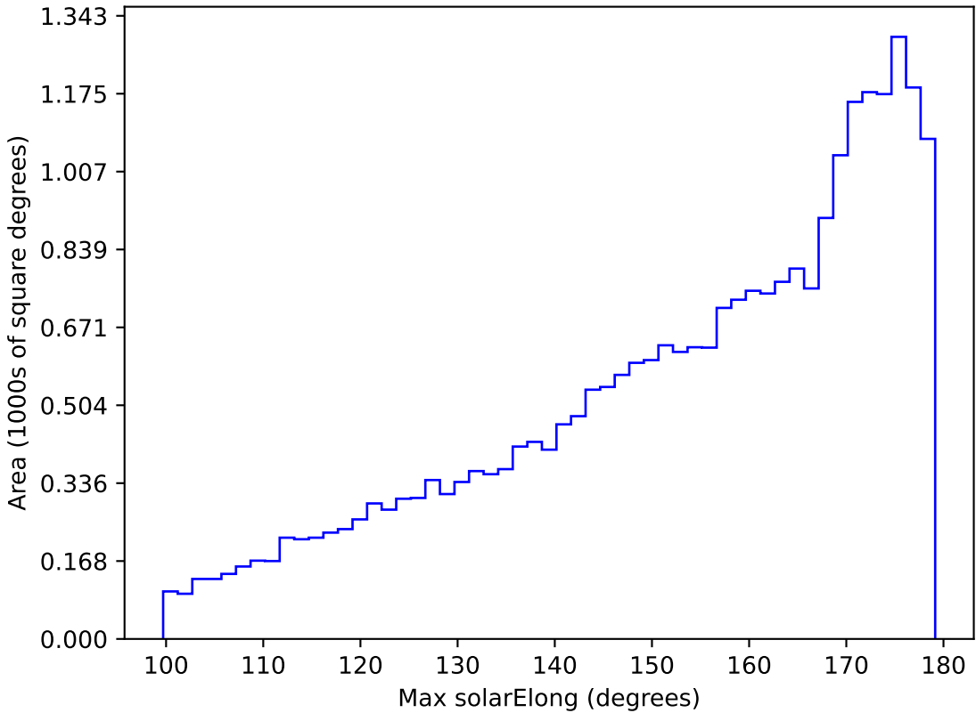
weather_cloudso6v3.4_10yrs All sky g band: Max solarElong
