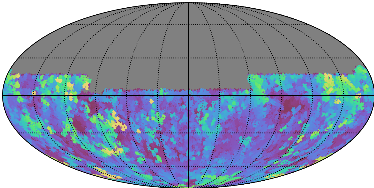
weather_cloudso6v3.4_10yrs Yr 1 y band: Max seeingEff
