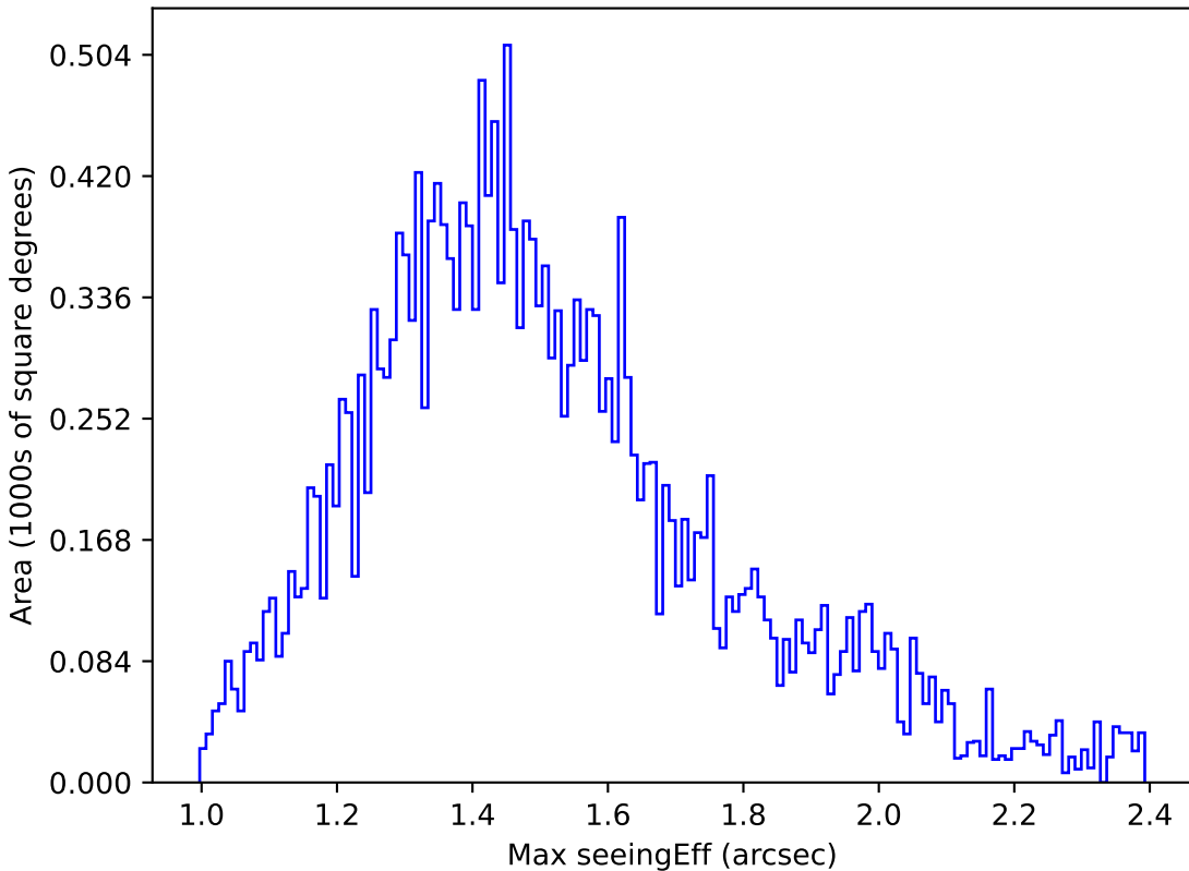
weather_cloudso6v3.4_10yrs Yr 1 y band: Max seeingEff
