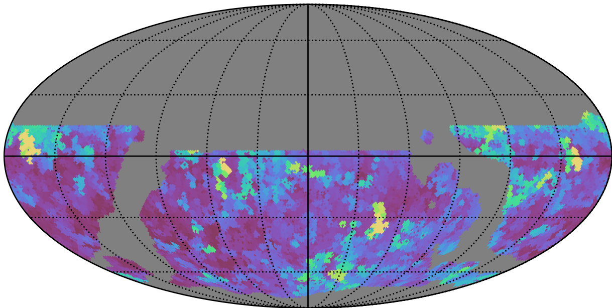
weather_cloudso6v3.4_10yrs WFD i band: Max seeingEff
