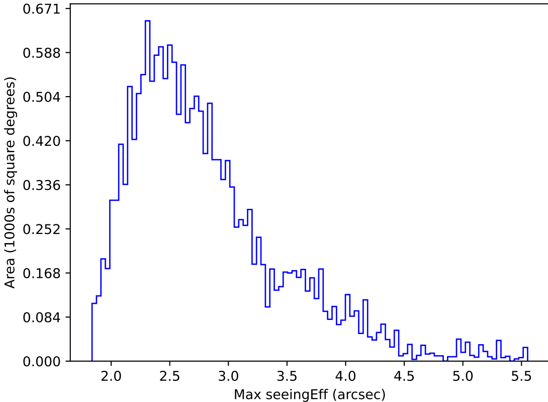
weather_cloudso6v3.4_10yrs WFD i band: Max seeingEff
