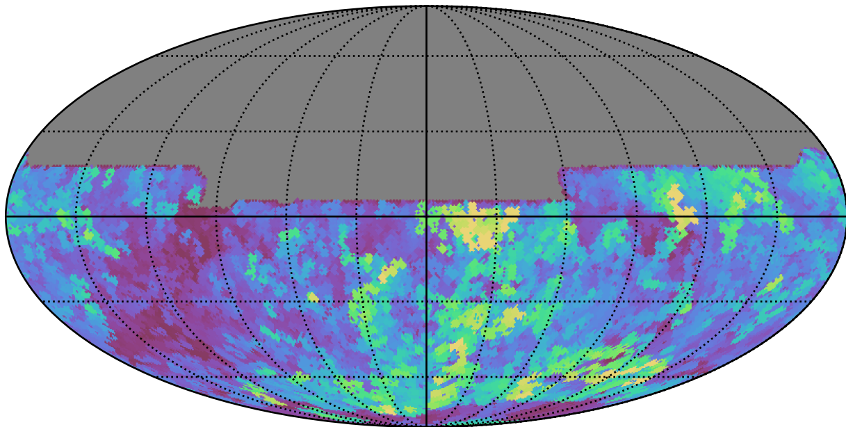
weather_cloudso6v3.4_10yrs All sky y band: Max seeingEff
