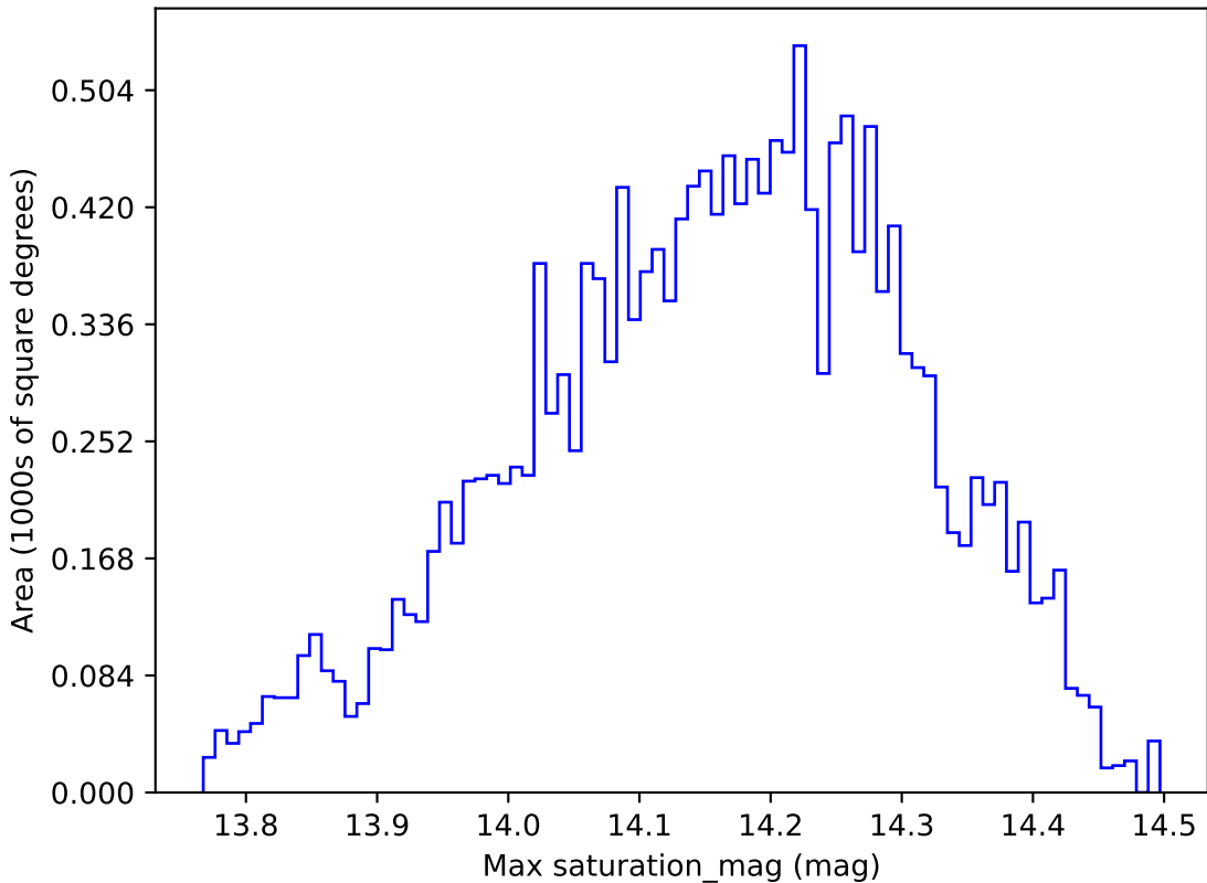
weather_cloudso6v3.4_10yrs WFD y band: Max saturation_mag
