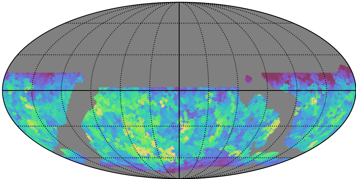
weather_cloudso6v3.4_10yrs WFD r band: Max saturation_mag
