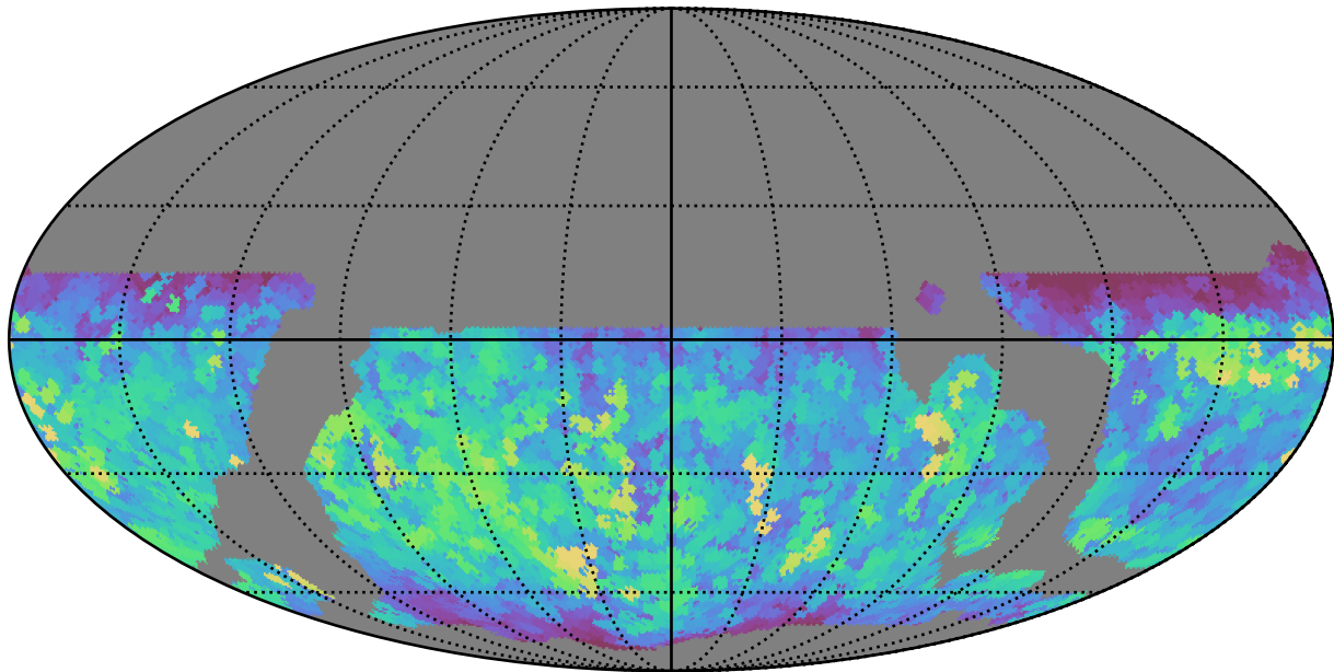
weather_cloudso6v3.4_10yrs WFD i band: Max saturation_mag
