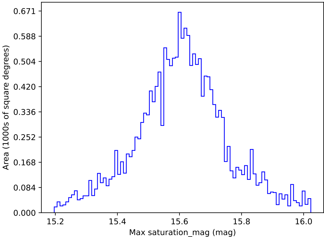
weather_cloudso6v3.4_10yrs WFD i band: Max saturation_mag
