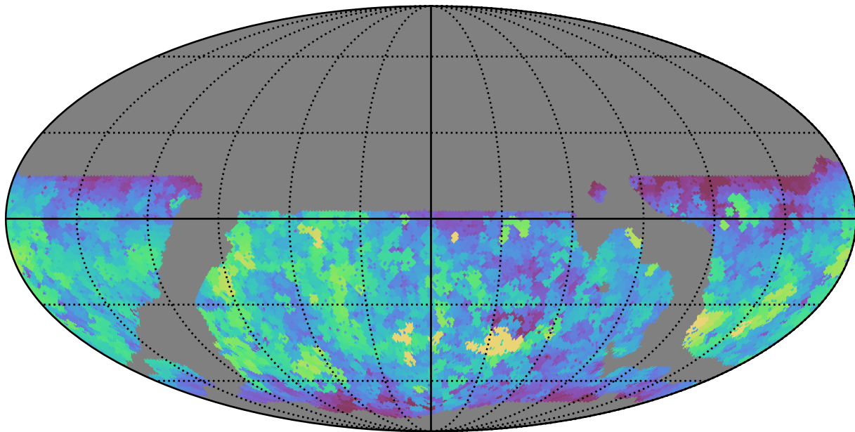
weather_cloudso6v3.4_10yrs WFD g band: Max saturation_mag
