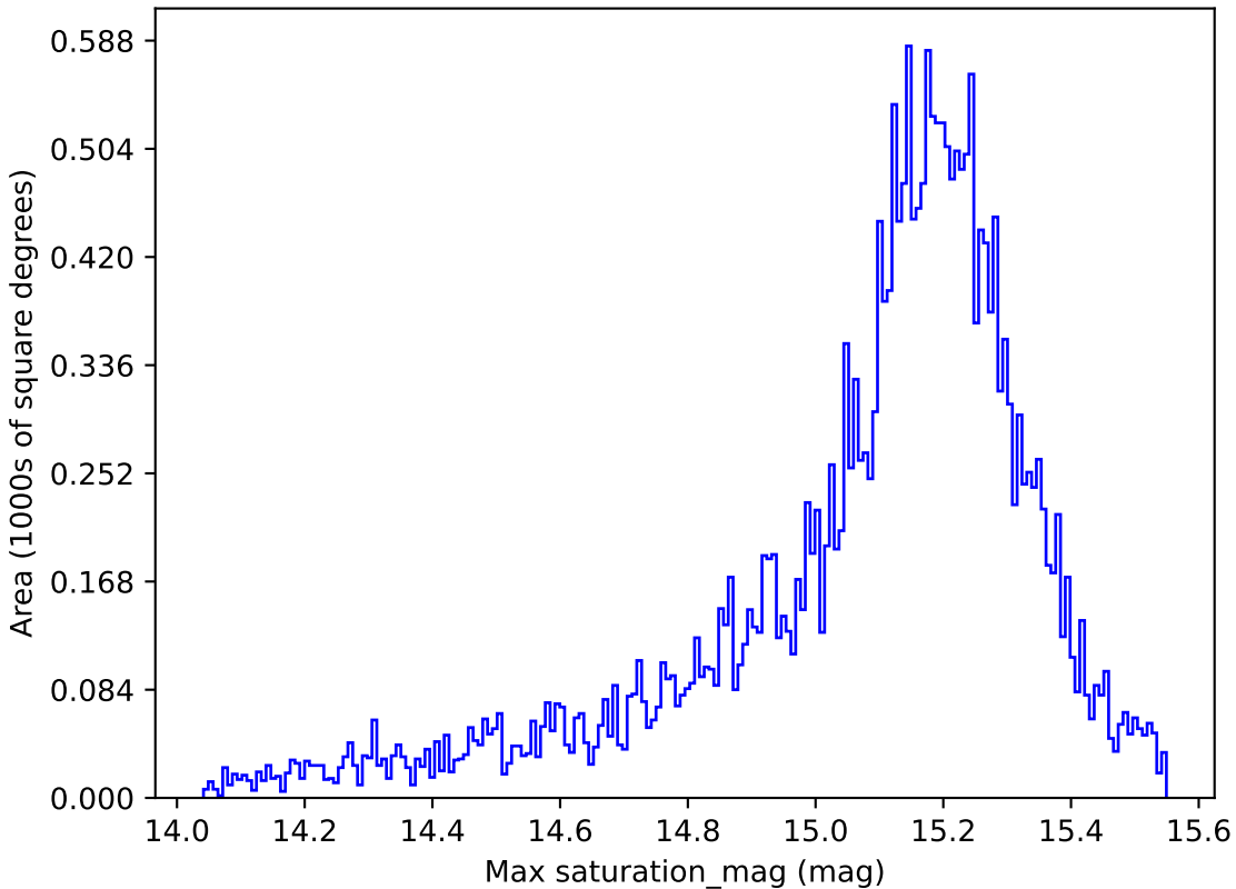
weather_cloudso6v3.4_10yrs All sky z band: Max saturation_mag
