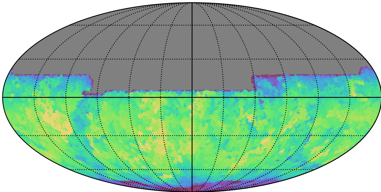
weather_cloudso6v3.4_10yrs All sky y band: Max saturation_mag
