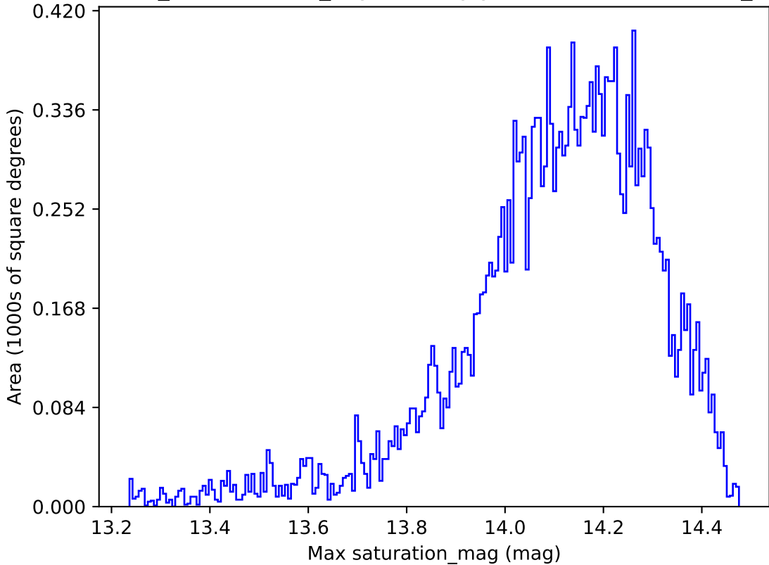
weather_cloudso6v3.4_10yrs All sky y band: Max saturation_mag
