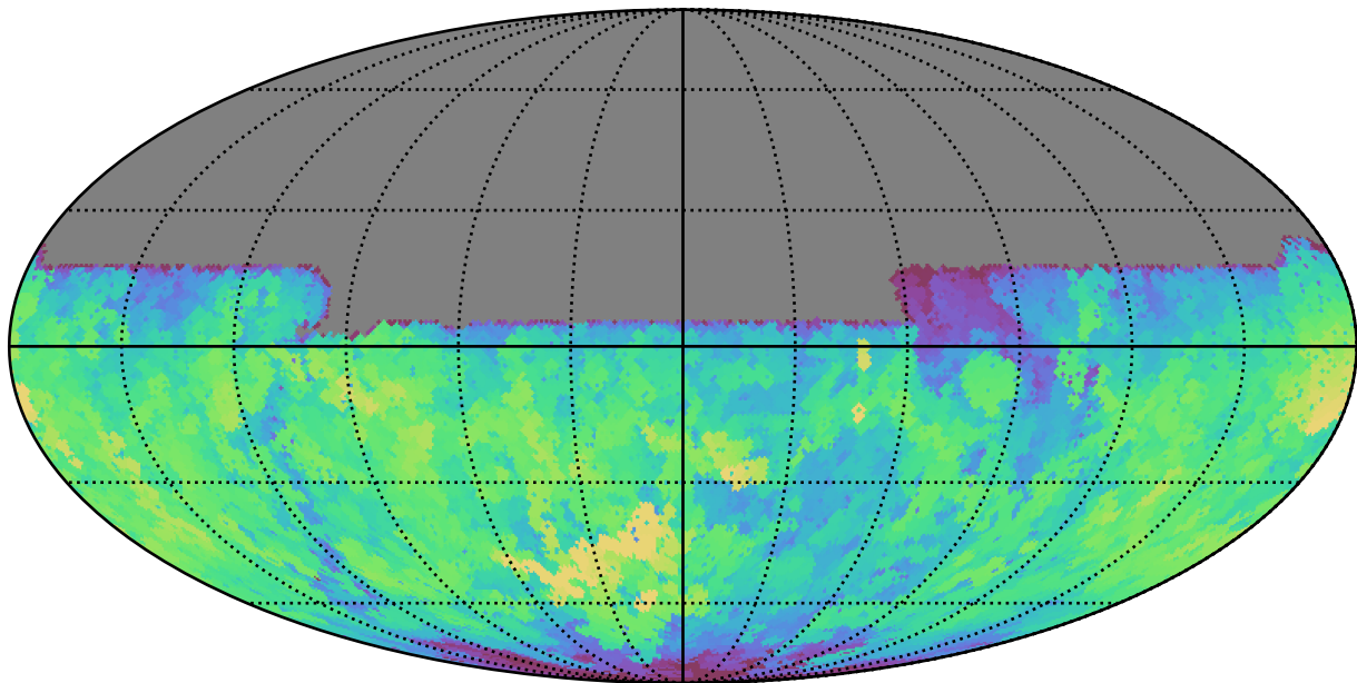
weather_cloudso6v3.4_10yrs All sky u band: Max saturation_mag
