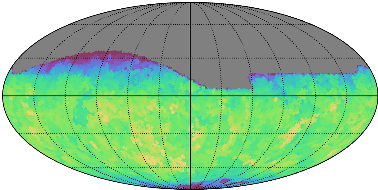
weather_cloudso6v3.4_10yrs All sky r band: Max saturation_mag
