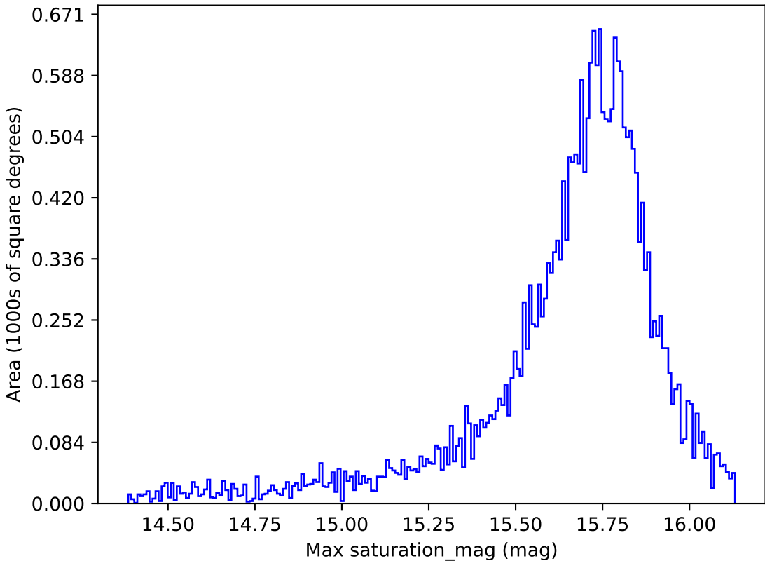
weather_cloudso6v3.4_10yrs All sky r band: Max saturation_mag
