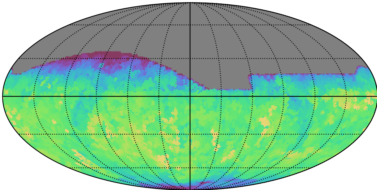
weather_cloudso6v3.4_10yrs All sky i band: Max saturation_mag
