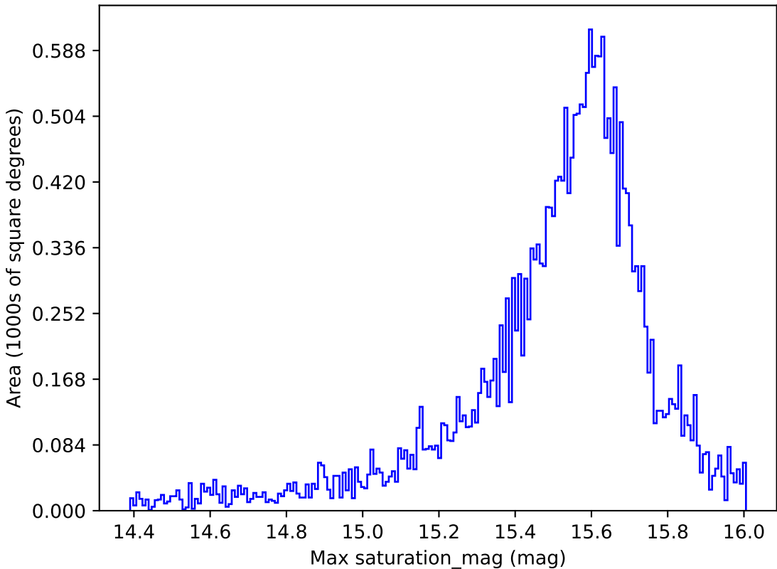
weather_cloudso6v3.4_10yrs All sky i band: Max saturation_mag
