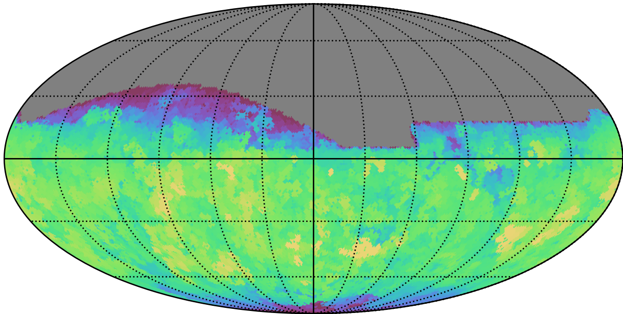
weather_cloudso6v3.4_10yrs All sky g band: Max saturation_mag
