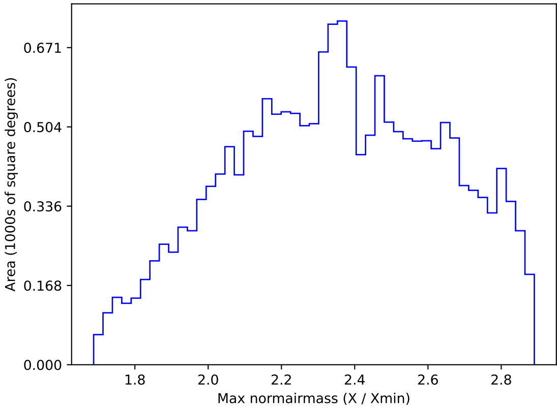
weather_cloudso6v3.4_10yrs WFD z band: Max normairmass
