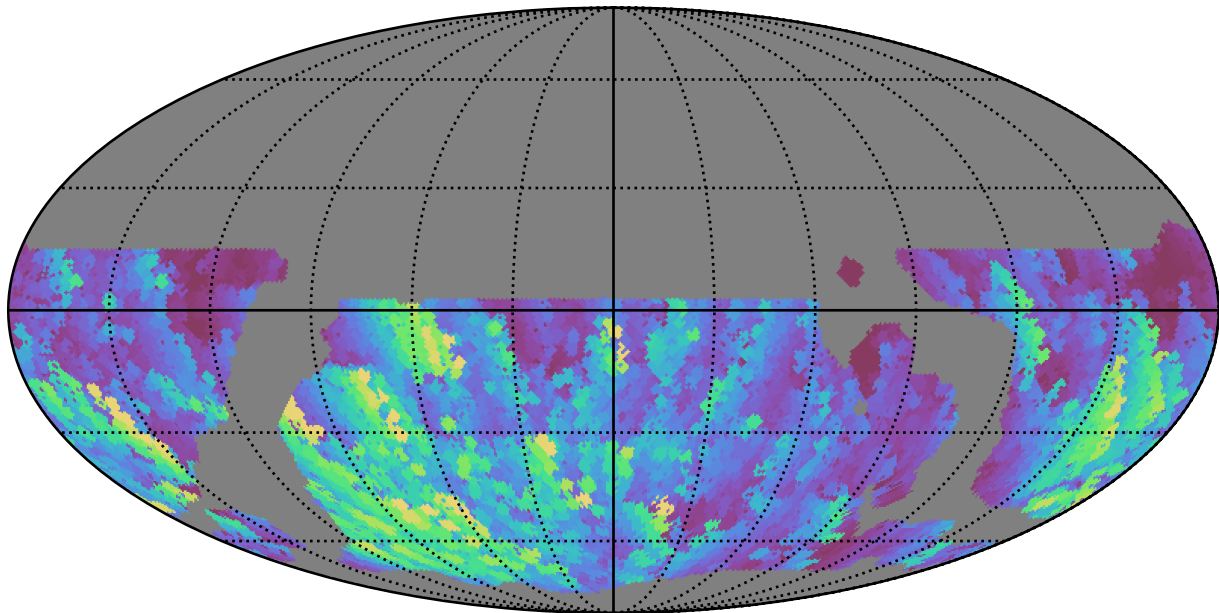
weather_cloudso6v3.4_10yrs WFD u band: Max normairmass
