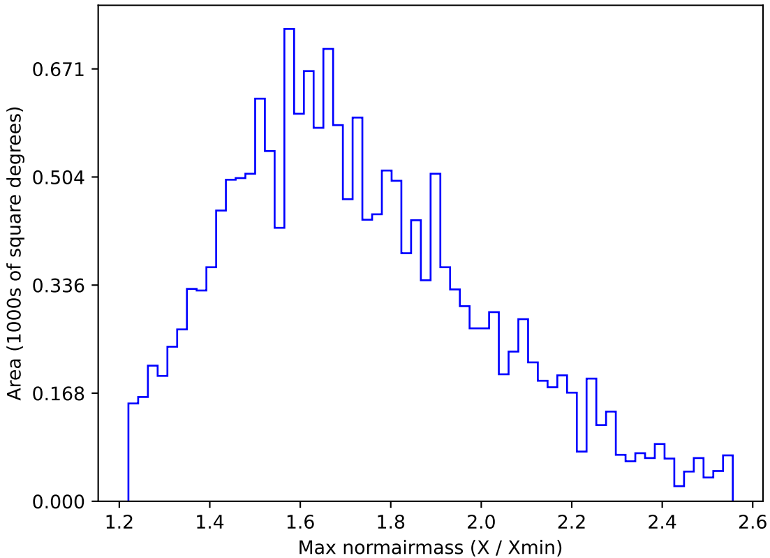
weather_cloudso6v3.4_10yrs WFD u band: Max normairmass
