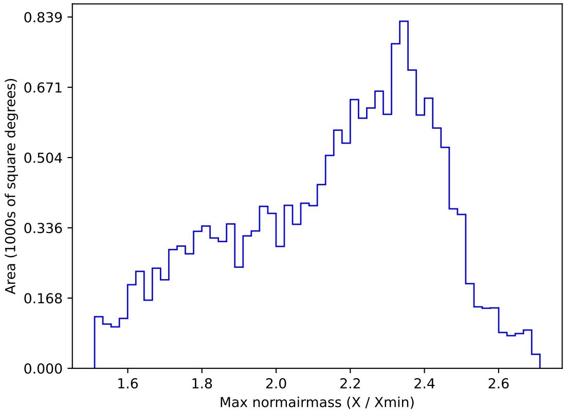
weather_cloudso6v3.4_10yrs WFD r band: Max normairmass
