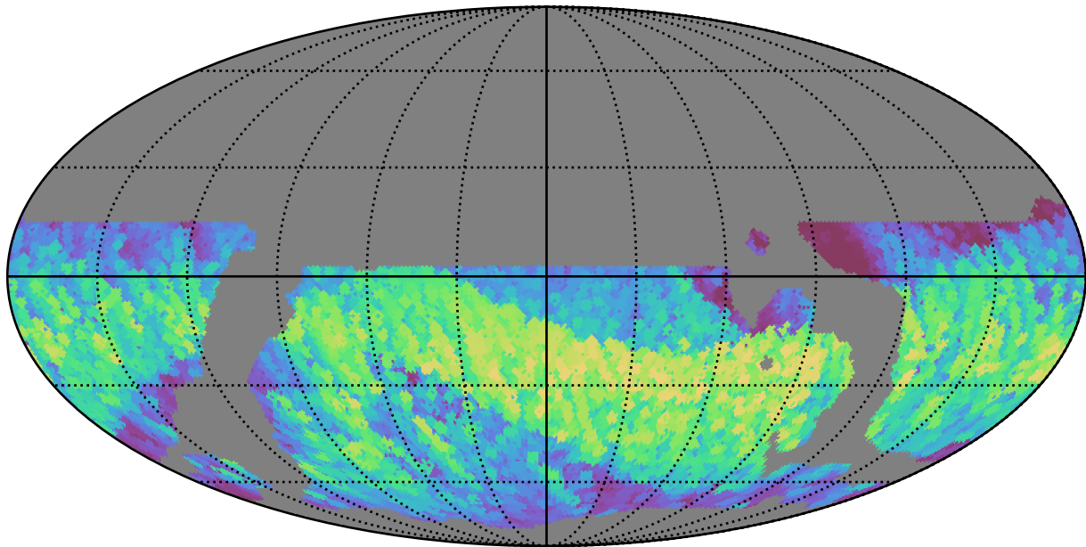
weather_cloudso6v3.4_10yrs WFD i band: Max normairmass
