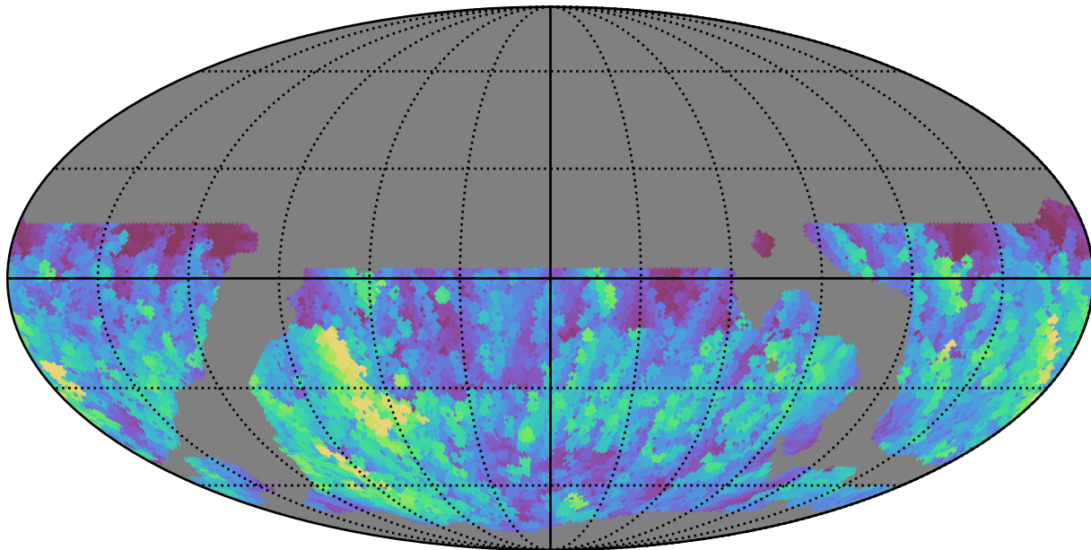
weather_cloudso6v3.4_10yrs WFD g band: Max normairmass
